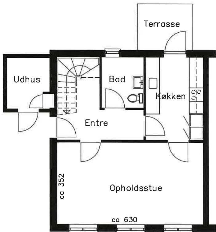
Stueplan
