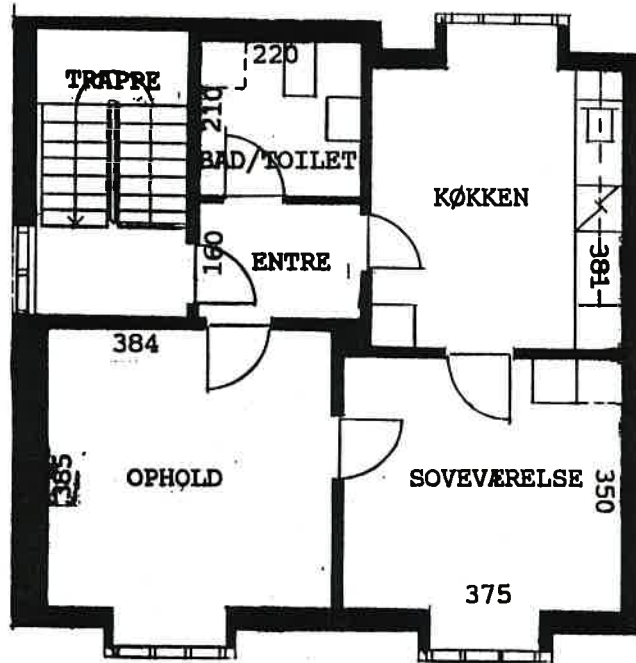
ETAGEPLAN
