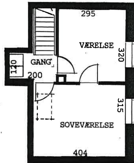
ETAGEPLAN
