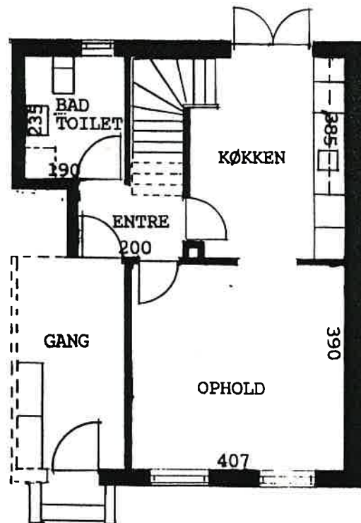
STUEPLAN
