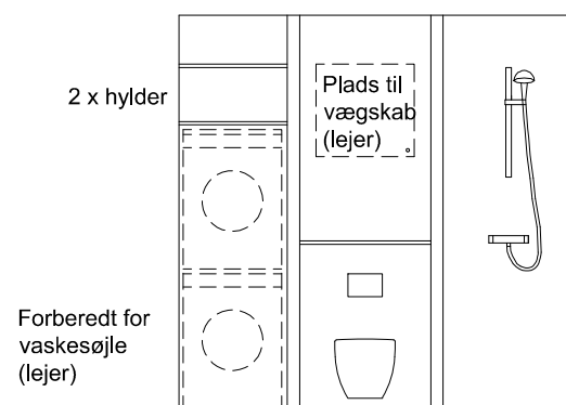
Opstalt af væg mod lejlighedsskel
