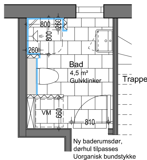
Dobbelthuse Stueplan - Forslag til nyt badeværelse
