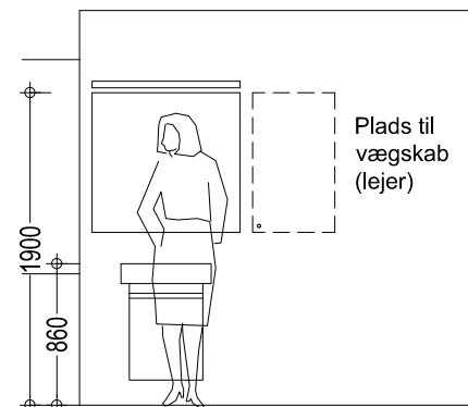
Opstalt af væg mod trappe
