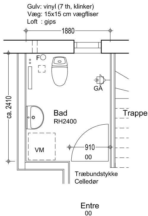
Dobbelthuse Stueplan - Eksisterende forhold
