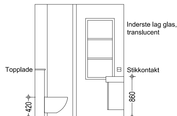
Opstalt af væg mod facade
