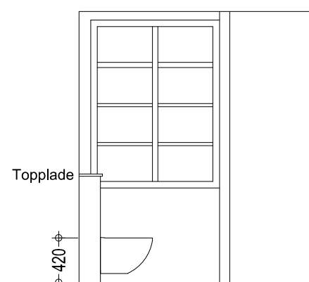
Opstalt af væg mod facade
