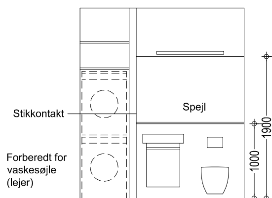
Opstalt af væg mod trappe
